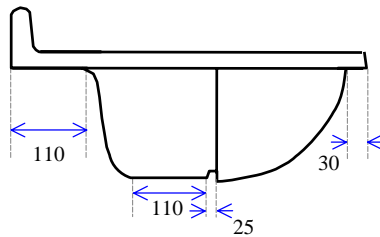
END ELEVATION
